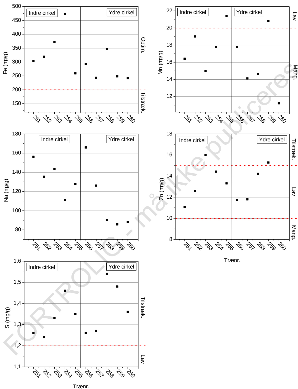
Figur 34: Koncentrationen af Fe, Mn, Na, Zn og S i bladprøver fra august, 2011. Diagnostiske koncentrationsintervaller: Optim.: optimal, Tilstræk.: Tilstrækkelig, Lav: lav og Mang.: Mangel.
