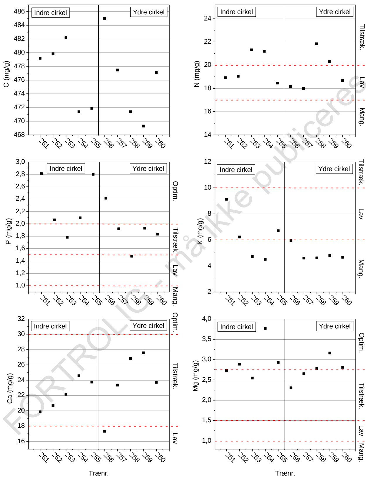
Figur 33: Koncentrationen af C, N, P, K, Ca og Mg i bladprøver fra august, 2011. Diagnostiske koncentrationsintervaller: Optim.: optimal, Tilstræk.: Tilstrækkelig, Lav: lav og Mang.: Mangel.
