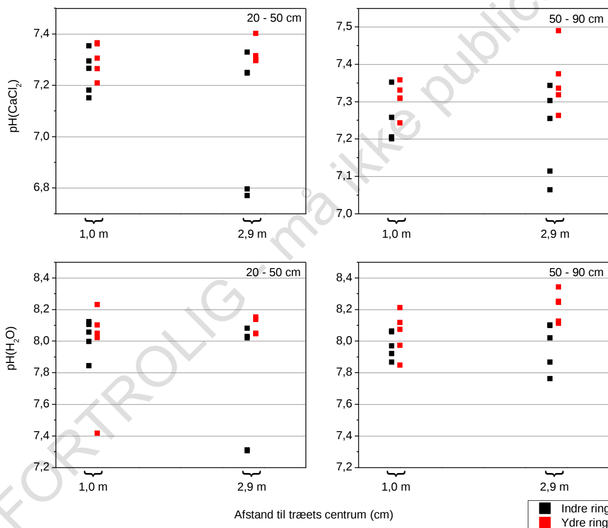
Figur 17: \text{pH}(\text{CaCl}_2) og \text{pH}(\text{H}_2\text{O}) i 40 jordbundsprøver fra Krinsen. Prøverne er taget i to forskellige afstande fra træerne (1,0 m og 2,9 m) samt fra to forskellige dybder under belægningens overkant (20 – 50 cm og 50 – 90 cm).
