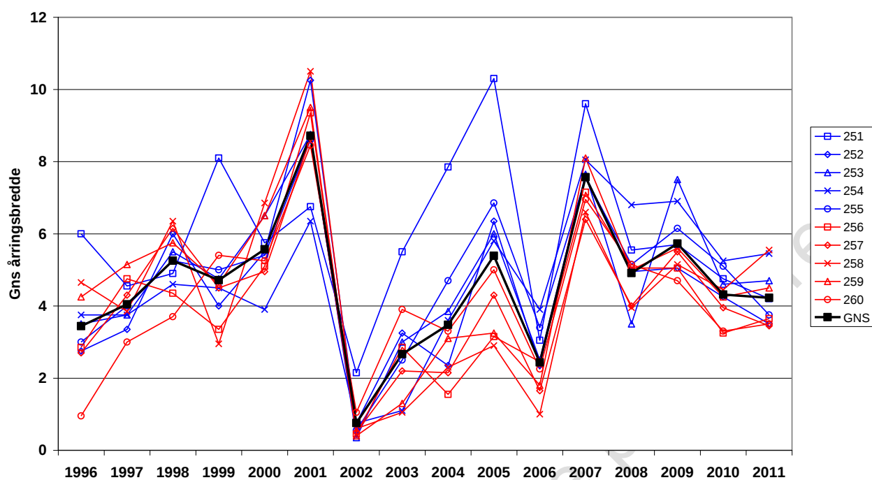
Figur 39: Gennemsnitlig årringsbredde for hvert træ, samt for alle ti træer (sort streg).
