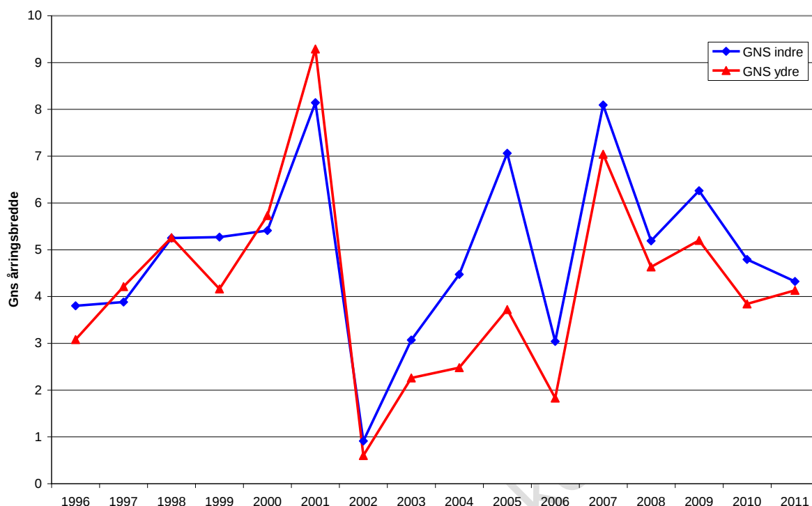
Figur 41: Gennemsnitlig årringsbredde for de ti måletræer opdelt på, om de stod i den indre (blå linje) eller ydre ring (rød linje). Før udplantning varierede årringsbredderne tilfældigt (se figur 35), men efter udplantning havde træerne i den indre ring i de fleste år en bedre diametervækst end træerne i den ydre ring.
